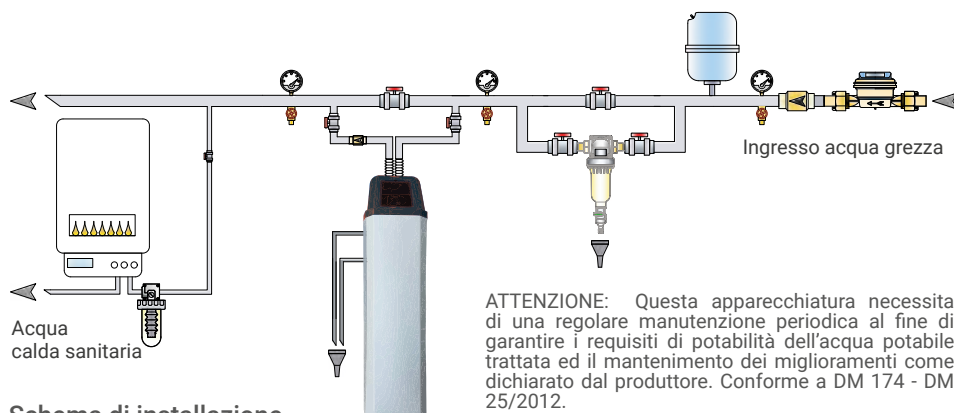
Schema di installazione
